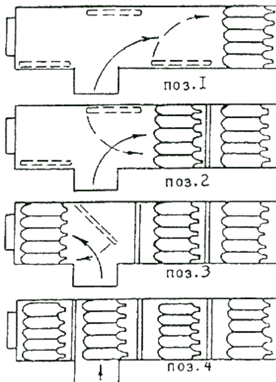
Вантаження тварин через бокові двері - трап з естакади
