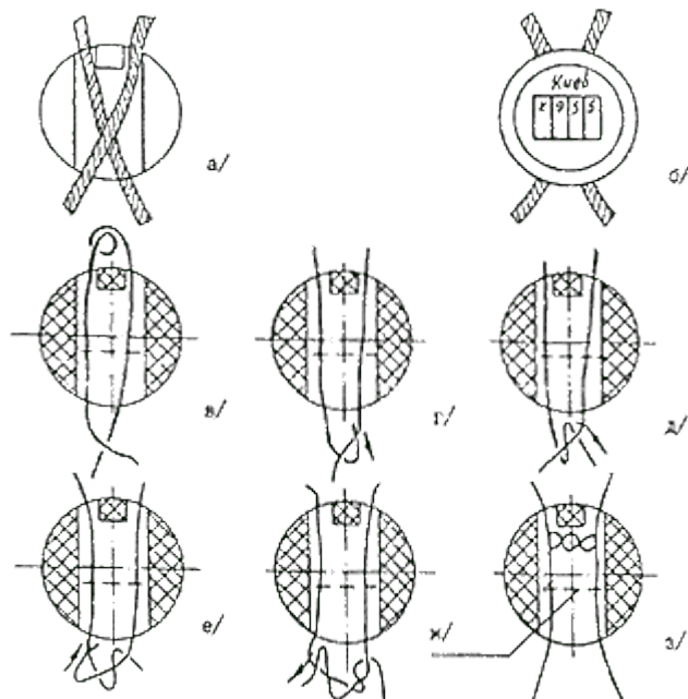
Способи навішування свинцевих (а, б) та поліетиленових (в - з) пломб із камерою
