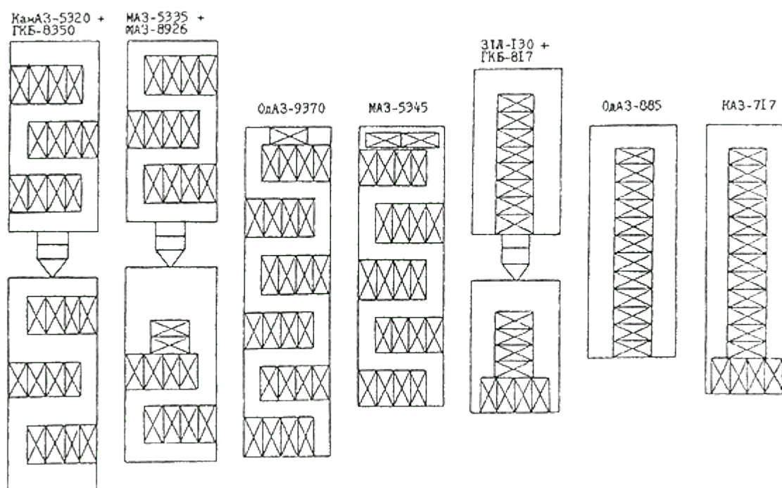
Схеми розміщення піддонів з цеглою на рухомому складі
