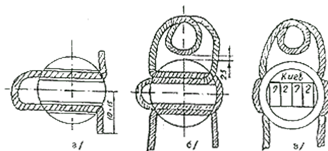
Способи навішування свинцевих (а, б) та поліетиленових (в - з) пломб із камерою
